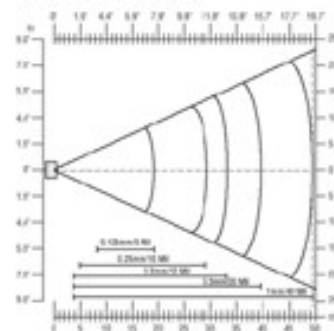
WDT2200 Laser
